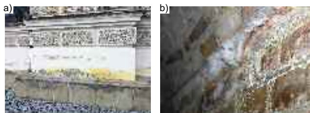
Przykład zawilgoconia kapilarnego (a) i wysoleń na konstrukcji murowej (b)
